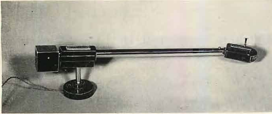
Fig. 2. Connoisseur magnetic pickup and arm.
